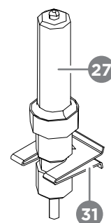
dettaglio A
